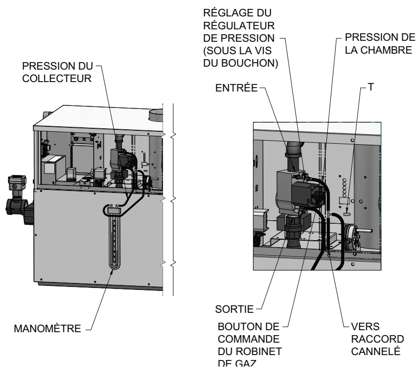
Figure 3-4_Mesure de la pression de gaz du collecteur
