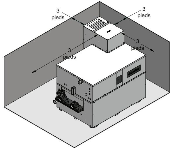
Figure 2-8 _Chapeau extérieur de ventilation installé sur les modèles 987 - 2067
