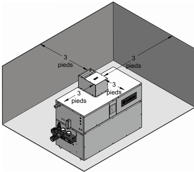
Figure 2-7 _Chapeau extérieur de ventilation installé sur les modèles 497 - 747
