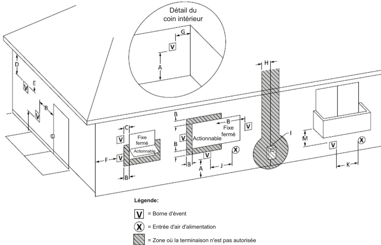
Figure 2-6 Autres que les espaces de terminaison de ventilation directe
